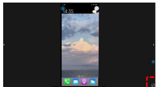
Vollbildanzeige
