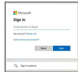
Anmeldungs-bildschirm (OneDrive)
