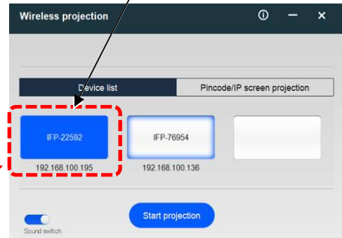
Windows-Bildschirm
